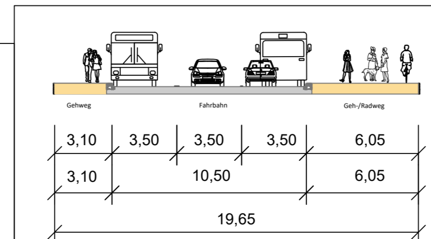
Regelquerschnitt A - A
