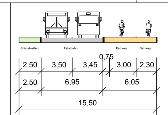
Regelquerschnitt B - B
